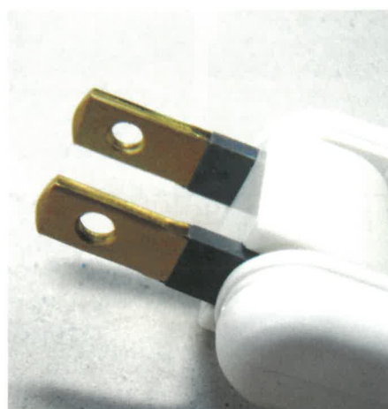
トラッキング防止被覆付き プラグもある
